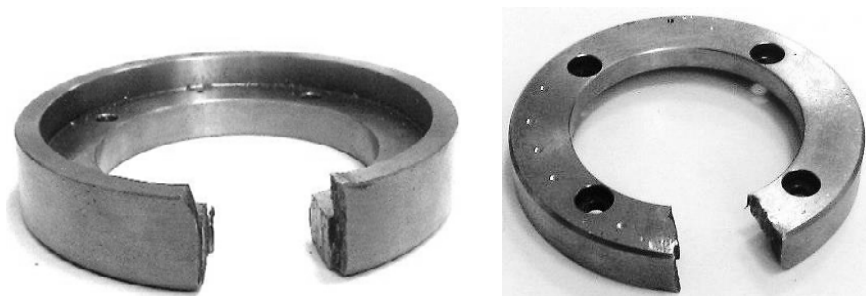
Рисунок 1 – Исследуемая деталь
