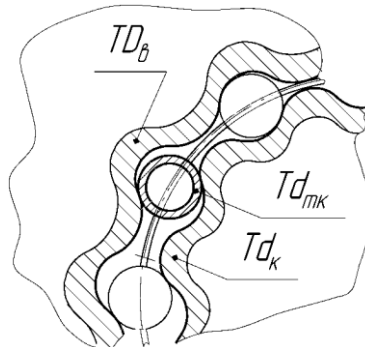
Рис. 2. Схема расположения допусков в зацепление передачи с ПТК и свободной обоймой.
