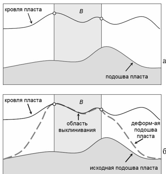
Рис. 1. Пример уточнения формы нефтяного пласта: а) до редактирования и б) после
